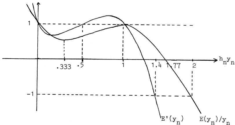
fig. 3.2. E(y_n)/y_n en E'(y_n) als functie van h_n y_n
