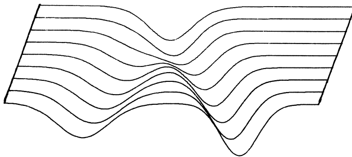
fig. 1.1 Epigenetisch landschap.
