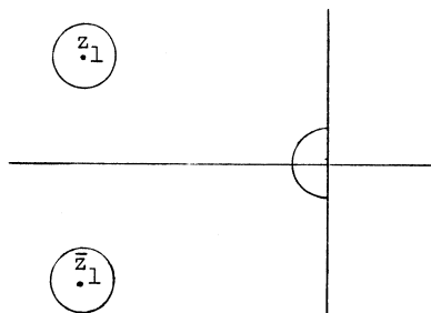
fig. 3.6. Stabiliteitsgebieden voor cluster-spectra
