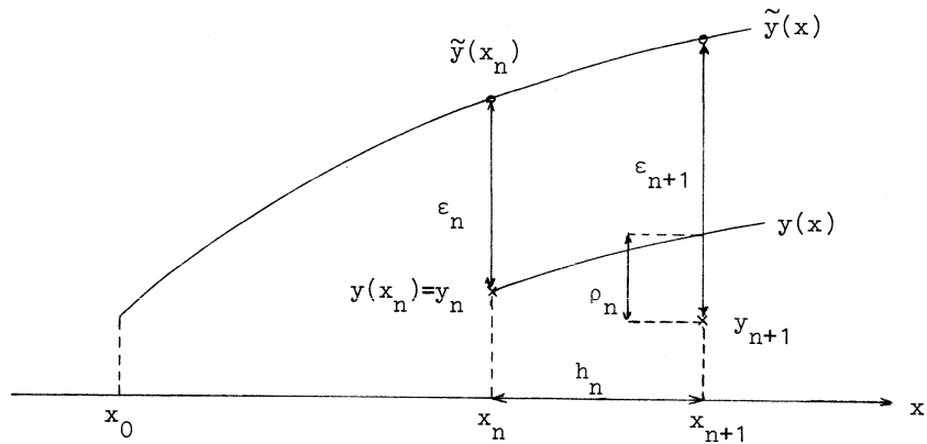
fig. 3.1. Illustratie van \rho_n en \epsilon_n
